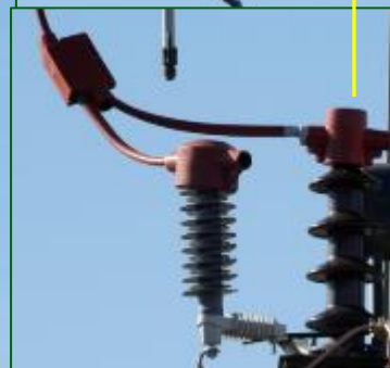
Mod. SPP : Protector para Aislador Rígido Polimérico 6704113 en uso como protector de Borna de Trafo.
