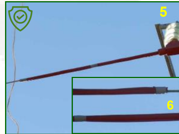
Imagen 5 : Encintado de seguridad del cierre mediante cinta de silicona autovulcanizable en frío , Mod. X-TREME de MOCAP®
