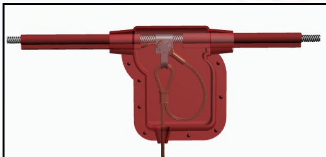
SPPD. Uso en Péndolas. Montaje de conjunto de forros modelos SPPD-SWP12-SWP28 .
