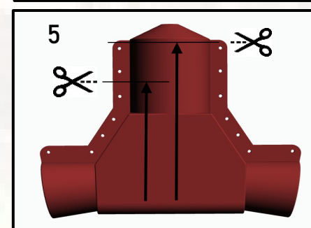
Montaje en Aisladores Poliméricos.
