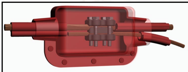
SPC. Uso en Empalmes Falso Sustentador. Montaje de conjunto de forros modelos SPC-SWP12-SWP28 .
