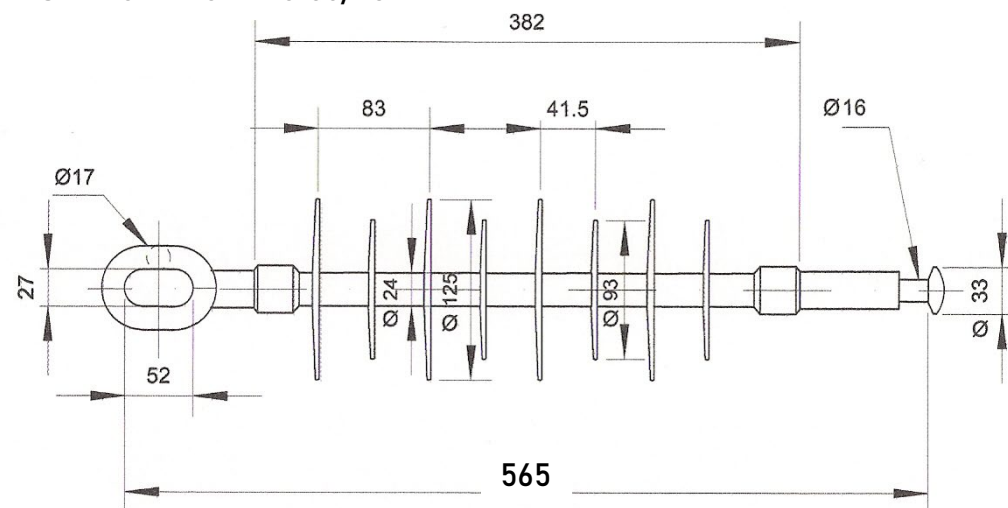
AISLADOR MODELO 36/70EB A
