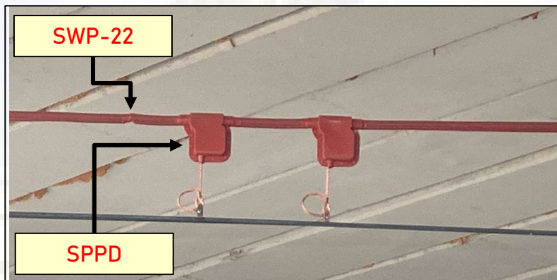
PROLONGACIÓN P.S. V21 SOBRE LA VÍA (PS 12+420)Tramo PB Alboraya - Massalfasar.
