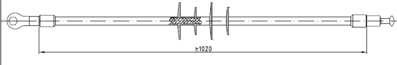
AISLADOR C3670YBAV_AR
