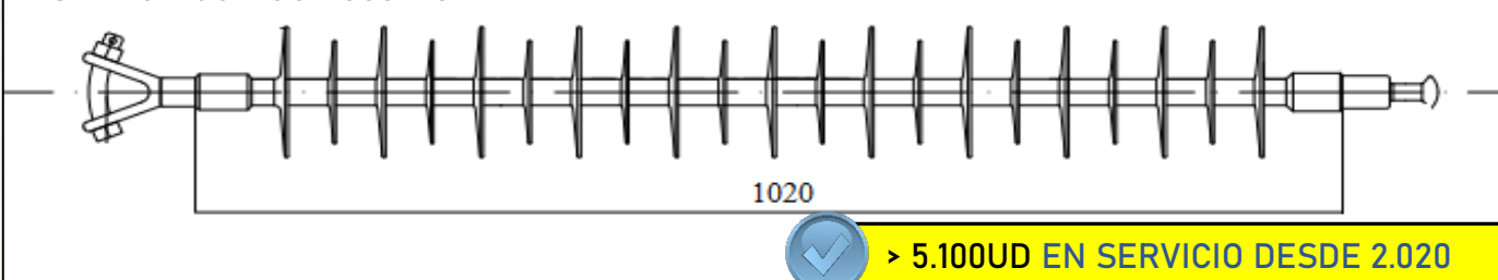
AISLADOR CÓDIGO 4803223
